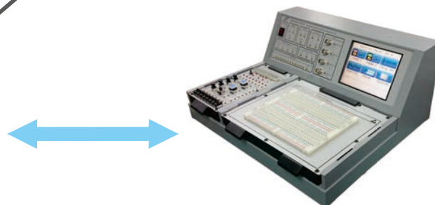
Пользовательский интерфейс
